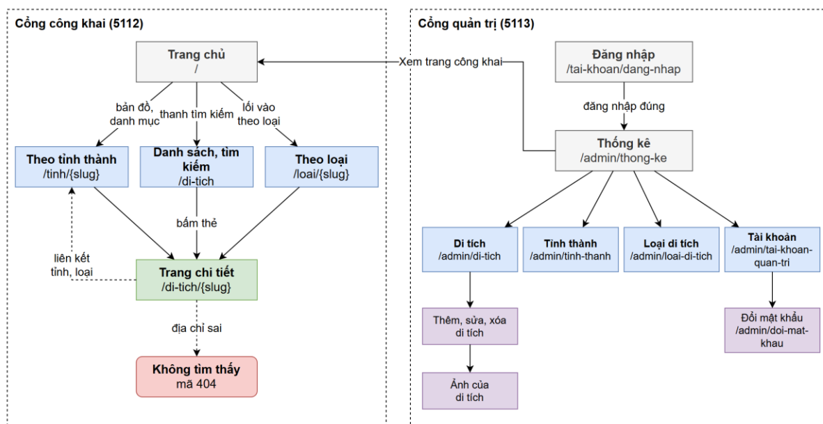
Sơ đồ 3.9. Sơ đồ điều hướng các trang
