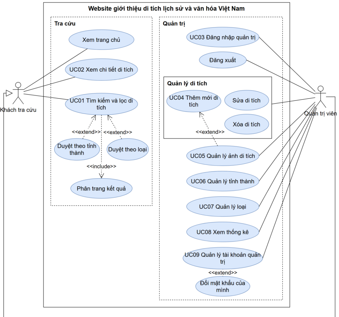
Sơ đồ 3.1. Sơ đồ use case tổng quát của hệ thống
