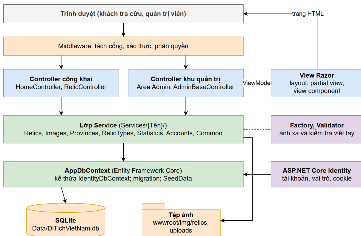
Sơ đồ 3.3. Kiến trúc phân lớp của hệ thống
