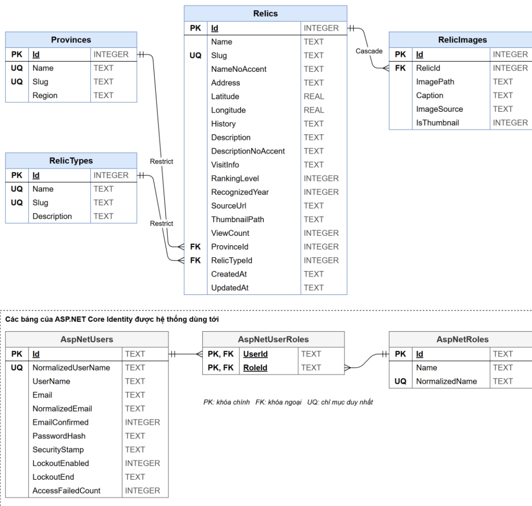
Sơ đồ 3.2. Sơ đồ thực thể liên kết của cơ sở dữ liệu
