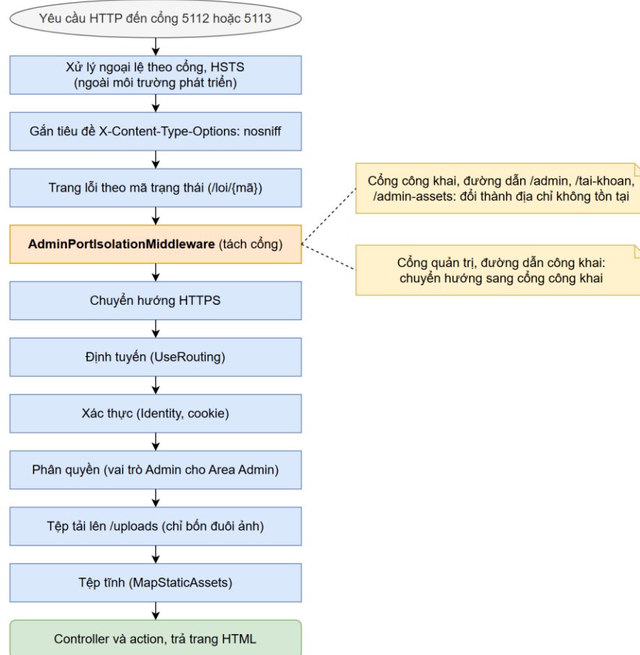
Sơ đồ 2.1. Đường ống middleware của ứng dụng
