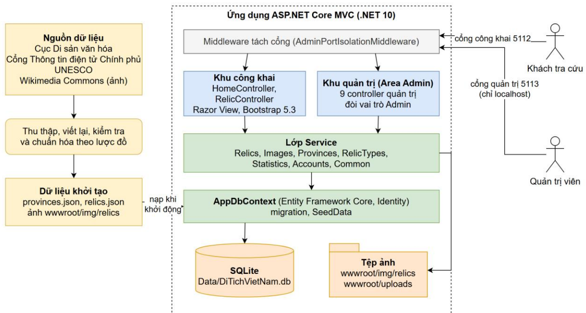
Sơ đồ 1.1. Sơ đồ tổng quan hệ thống
