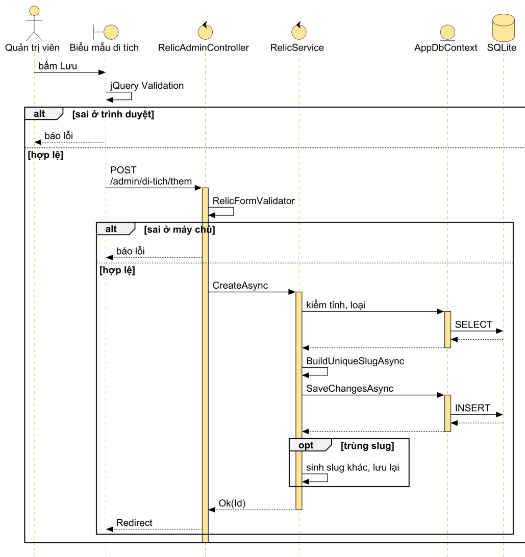
Sơ đồ 3.7. Sơ đồ tuần tự UC04 Thêm mới di tích
