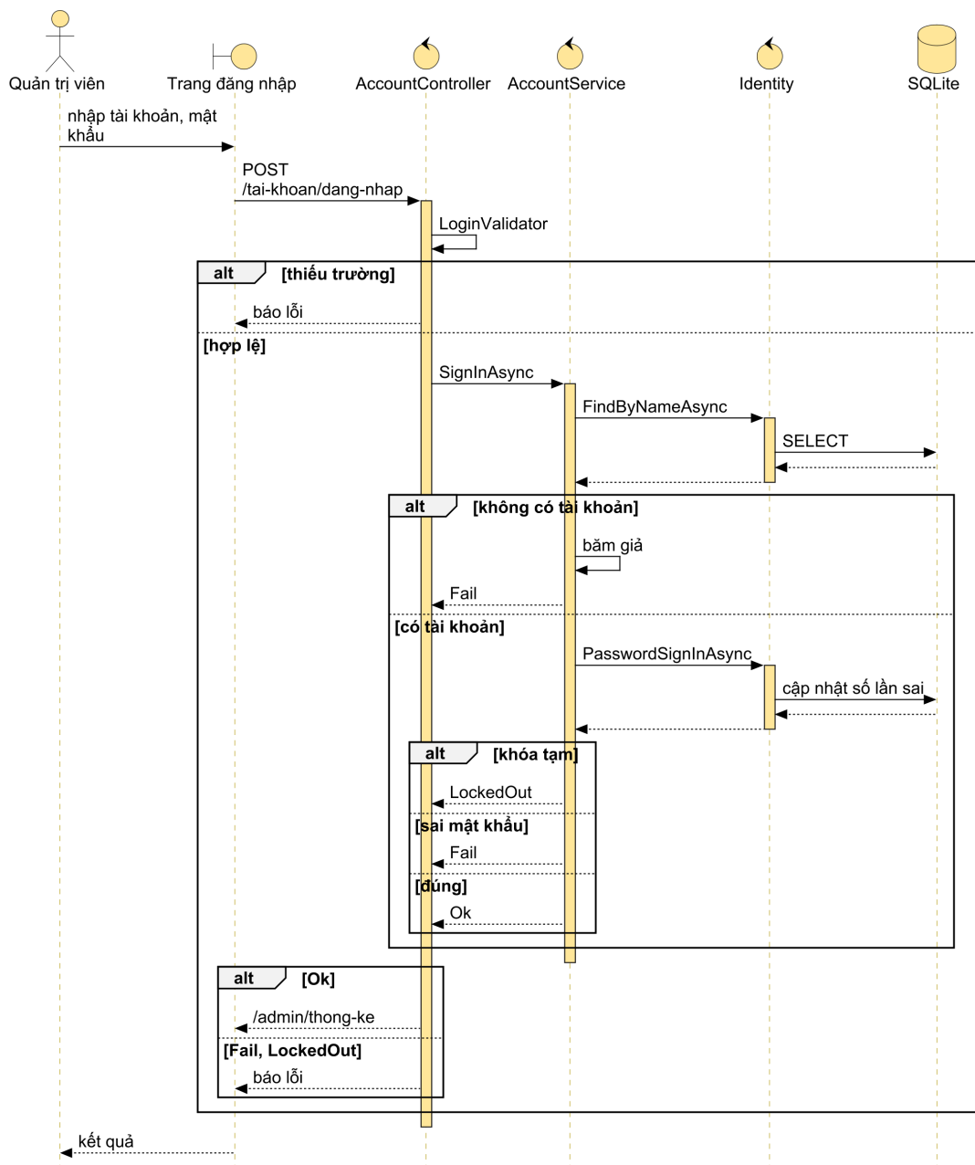
Sơ đồ 3.6. Sơ đồ tuần tự UC03 Đăng nhập quản trị
