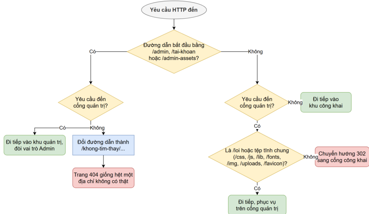
Sơ đồ 3.4. Đường đi của một yêu cầu qua middleware tách cổng
