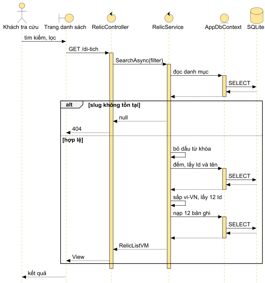
Sơ đồ 3.5. Sơ đồ tuần tự UC01 Tìm kiếm và lọc di tích
