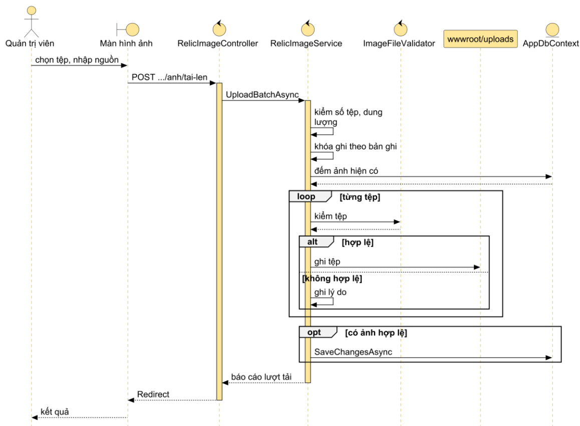
Sơ đồ 3.8. Sơ đồ tuần tự UC05 Quản lý ảnh di tích, thao tác tải nhiều ảnh
